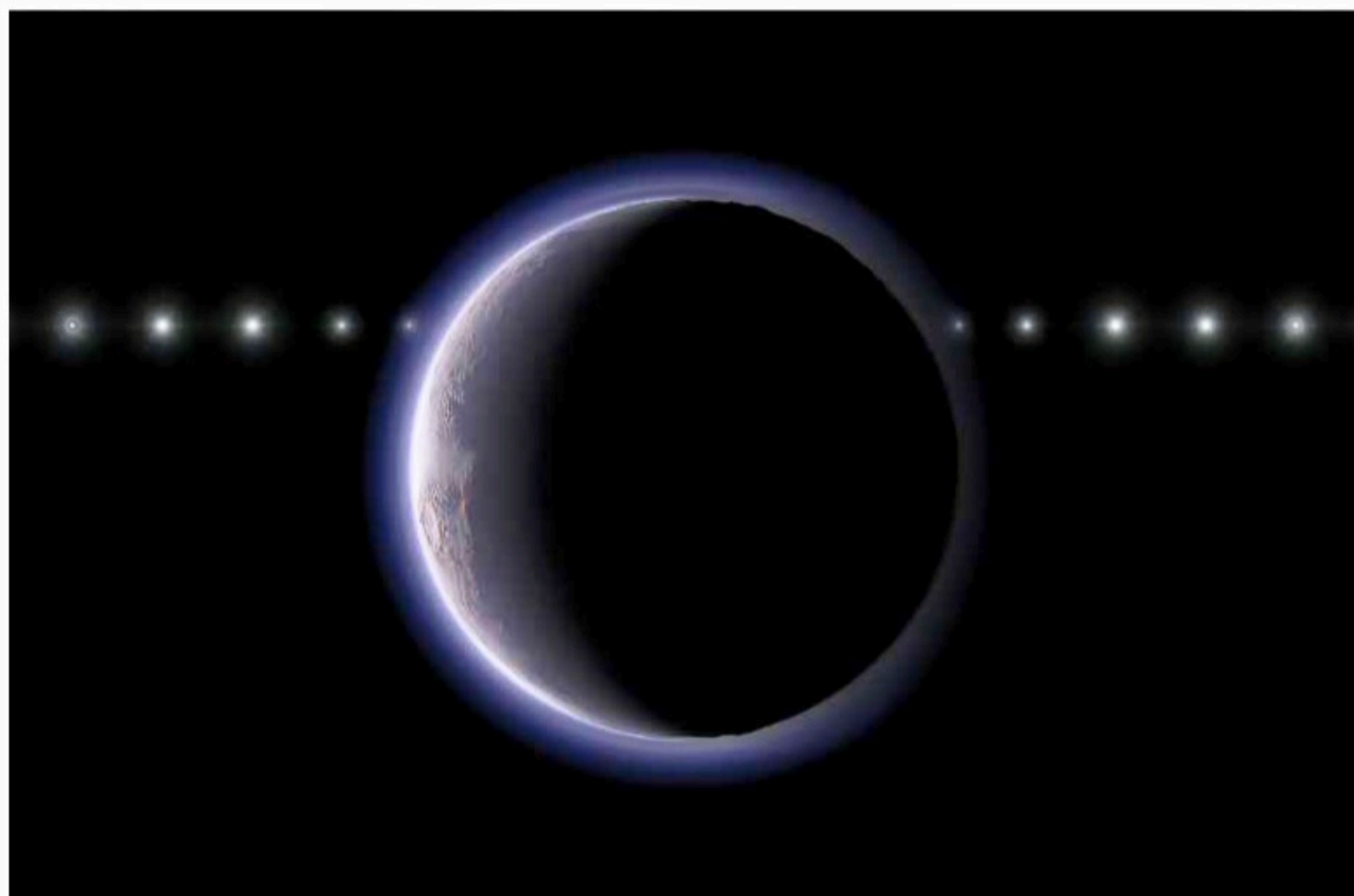
Ilustração do objeto batizado de (612533) 2002 XV93 Observatório Astronômico Nacional do Japão/Ko Arimatsu /AFP
